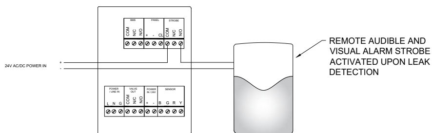
STROBE WIRING
