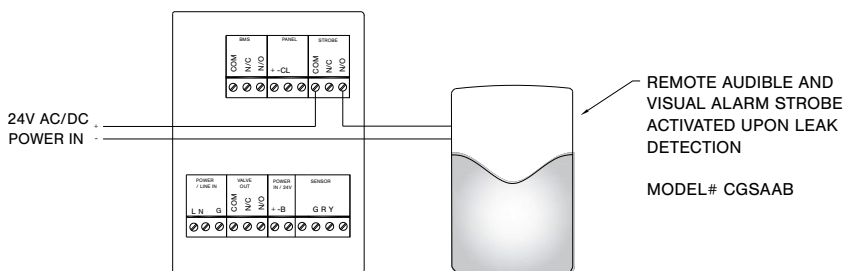
STROBE WIRING
