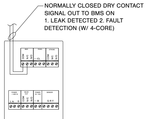
BMS WIRING
